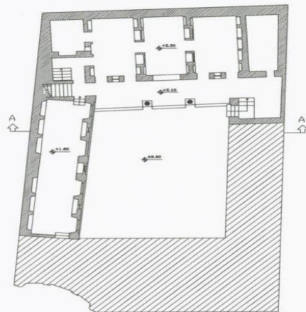
پلان طبقه اول
