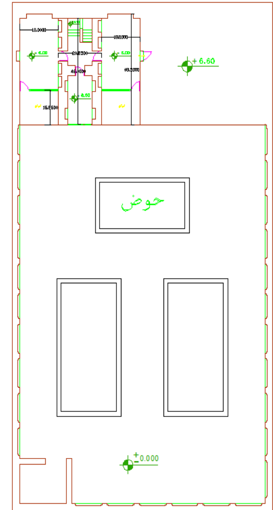
پلان طبقه دوم
