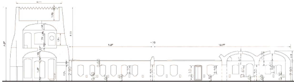
برش طولی برج و اصطبل ورودی
