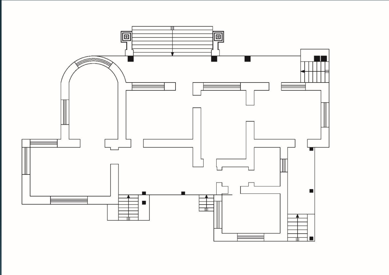
پلان طبقه همکف
