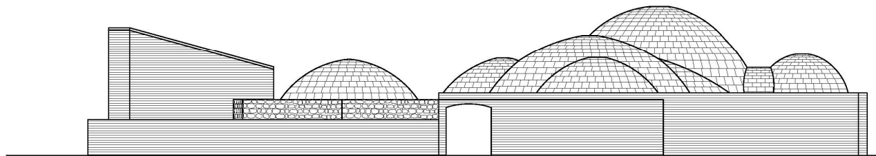
نمای غربی
