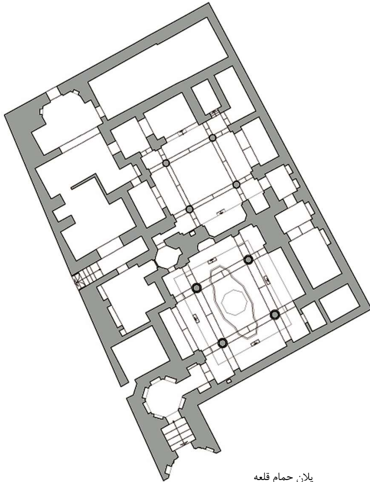
پلان حمام قلعه
